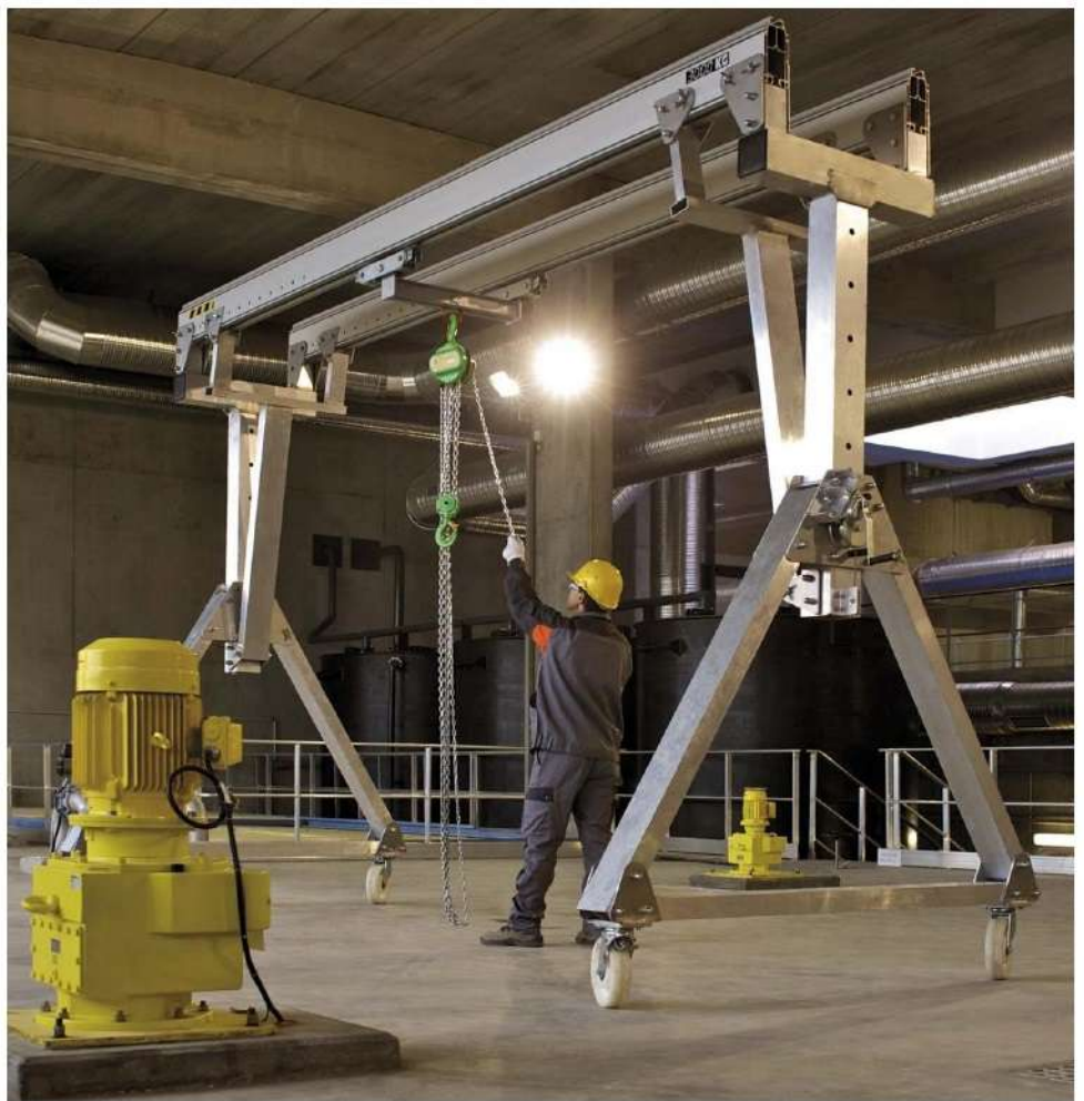
Diseño con perfil hueco para mayor flexibilidad
